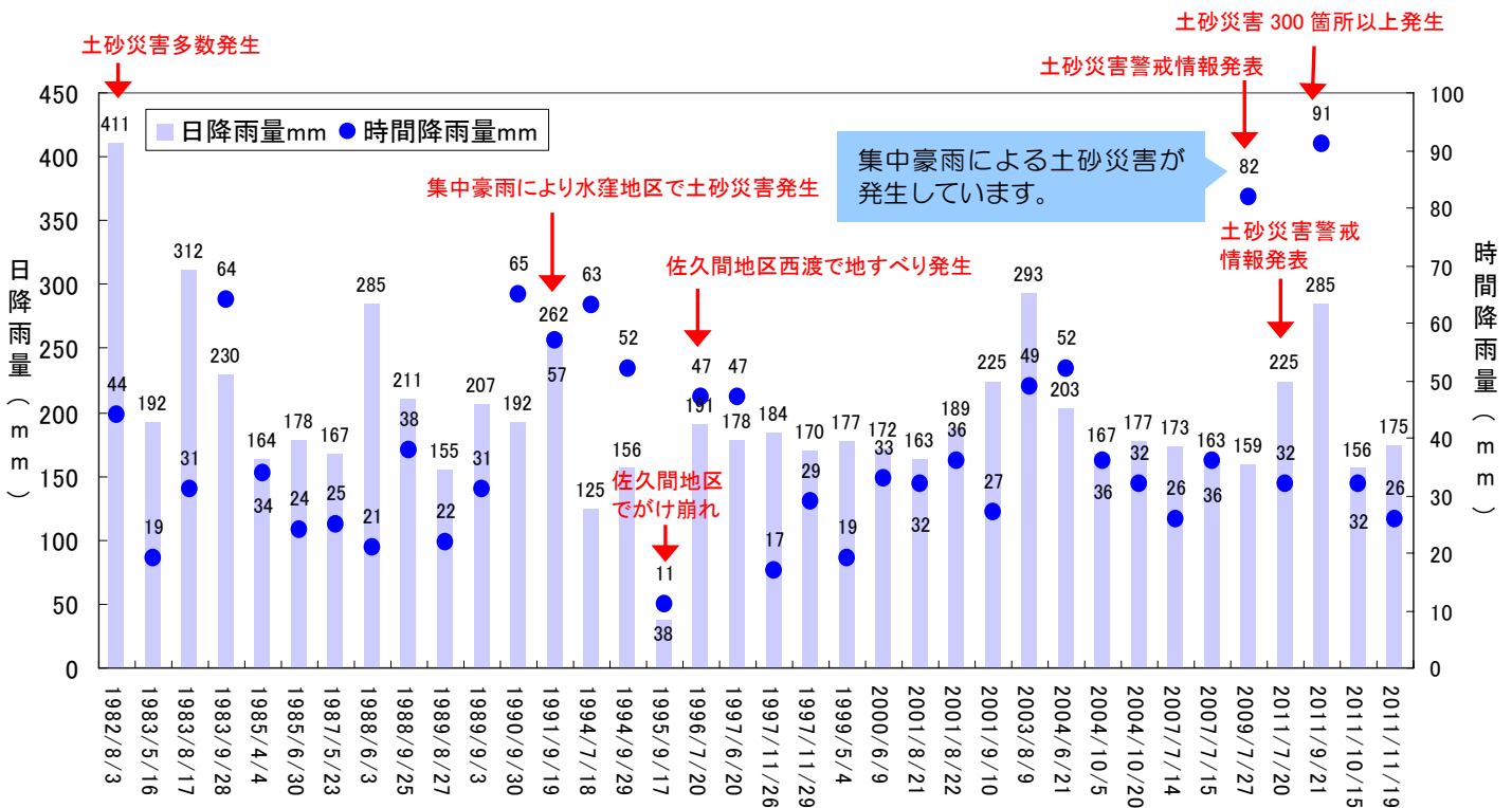
過去30年間の降雨量と土砂災害の傾向 (天竜区熊における日降水量150mm以上もしくは時間降水量60mm以上を抽出)
