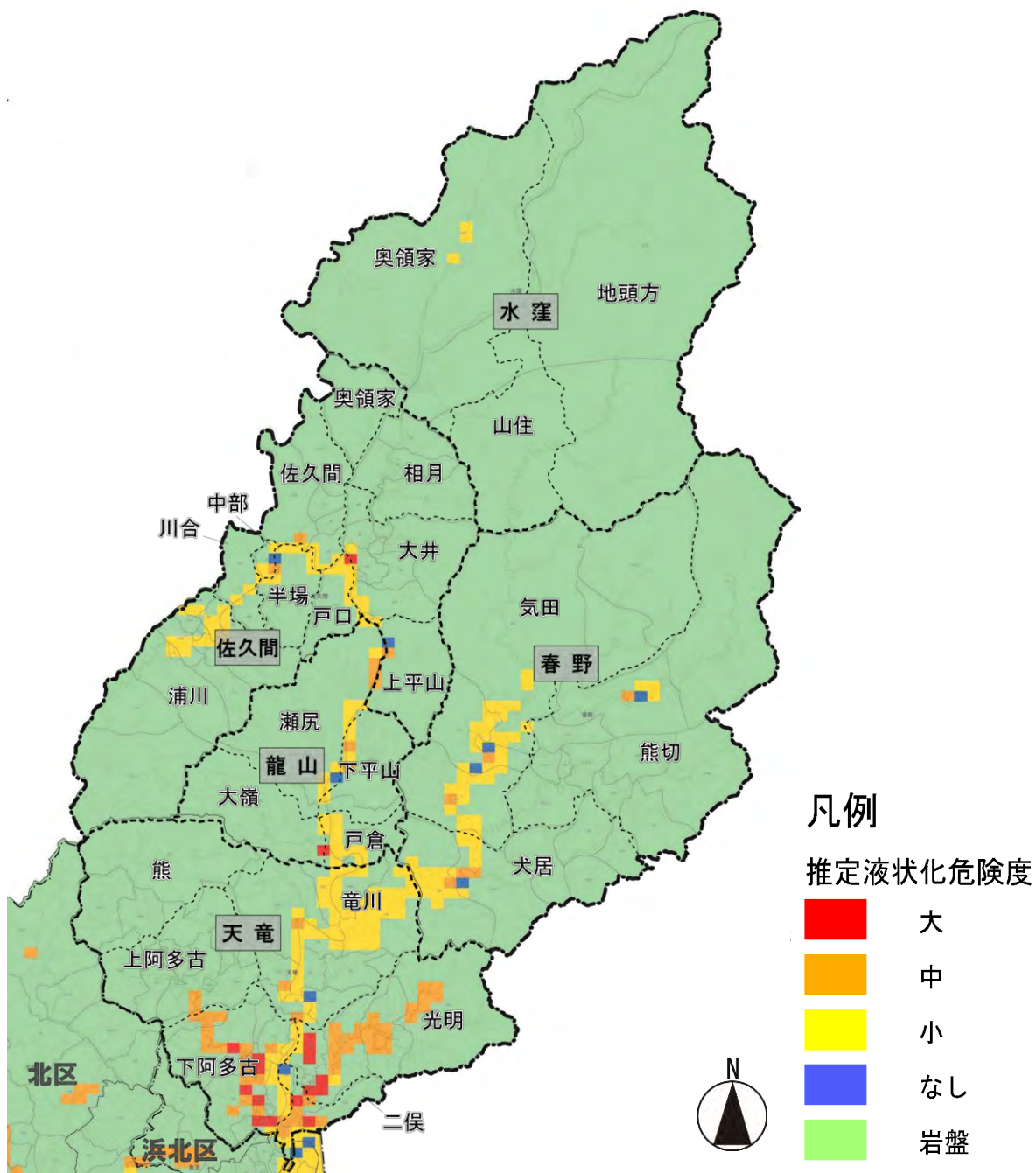
推定液状化危険度
