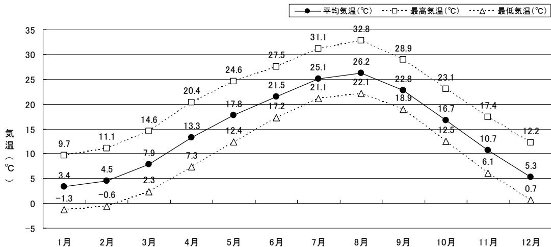
浜松市北部の月別気温（過去30年の平均、観測地点：佐久間）
