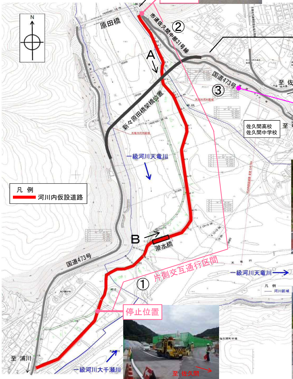
[河川内仮設道路平面図]
