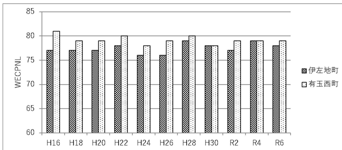
図 4-8 WECPNL による航空機騒音の経年変化(偶数年)
