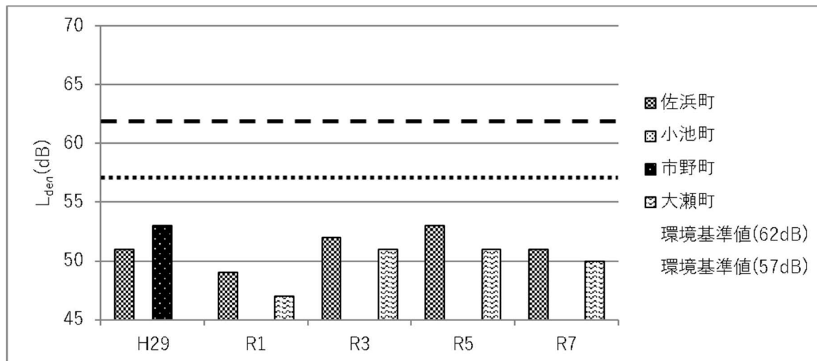
図 4-5 L_{den} による航空機騒音の経年変化(奇数年)
