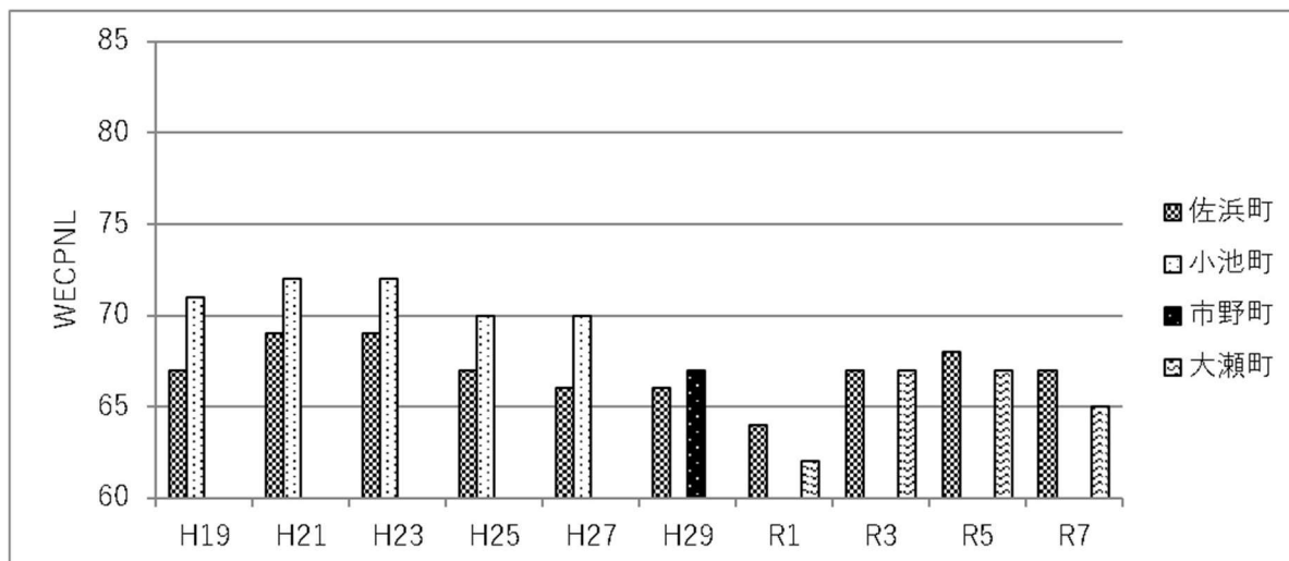
図 4-7 WECPNL による航空機騒音の経年変化(奇数年)
