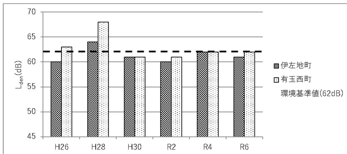
図 4-6 L_{den} による航空機騒音の経年変化(偶数年)
