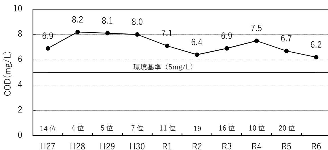
図 4 佐鳴湖の COD(年平均值)の経年変化
