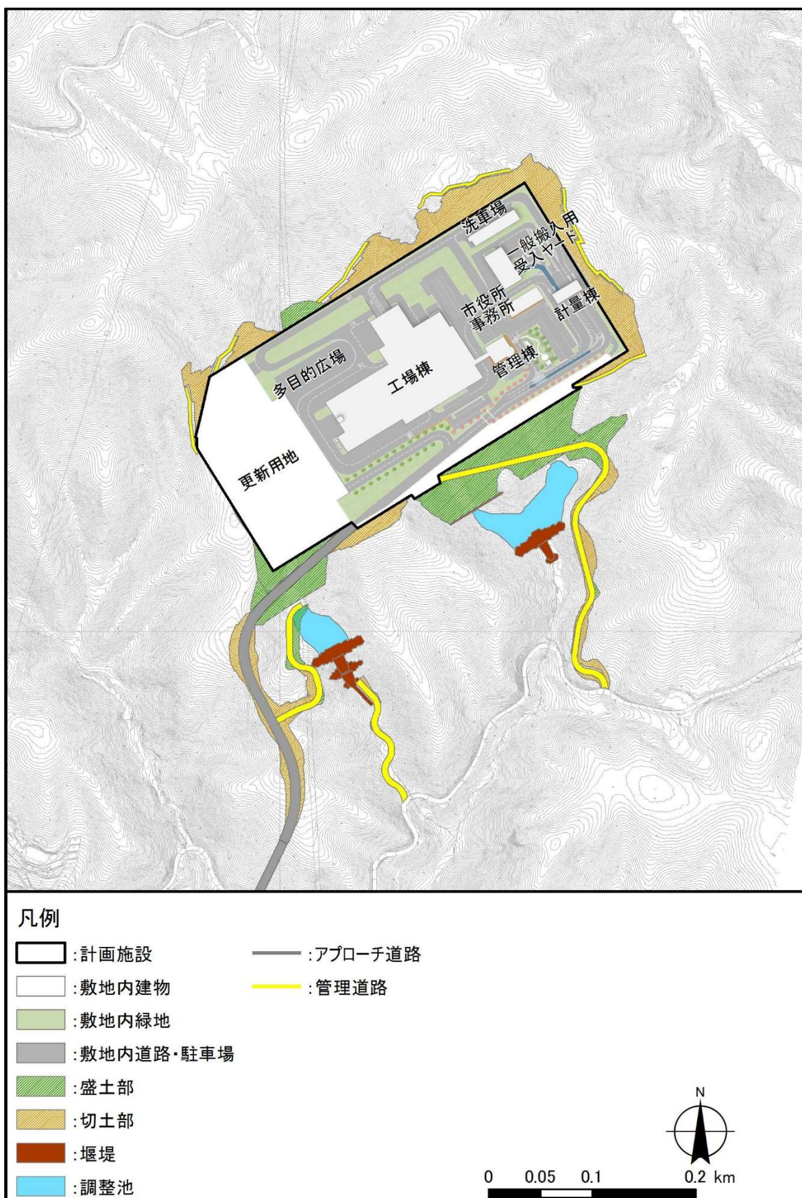
図 1-2 敷地造成及び施設配置計画
