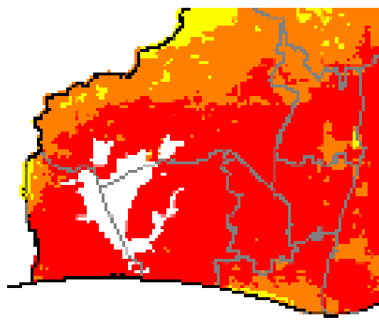
震度分布
