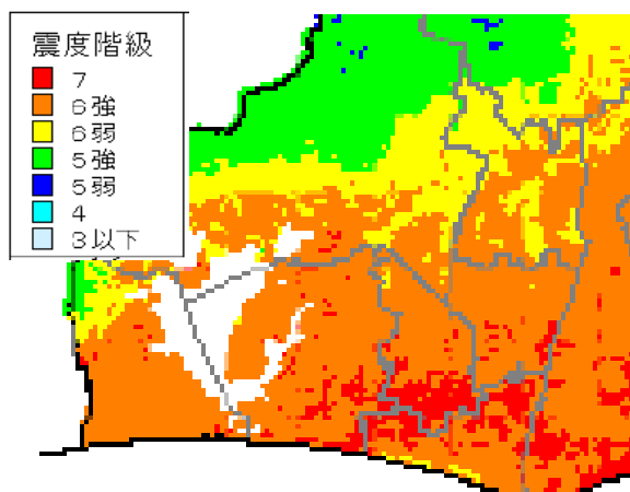
震度分布
