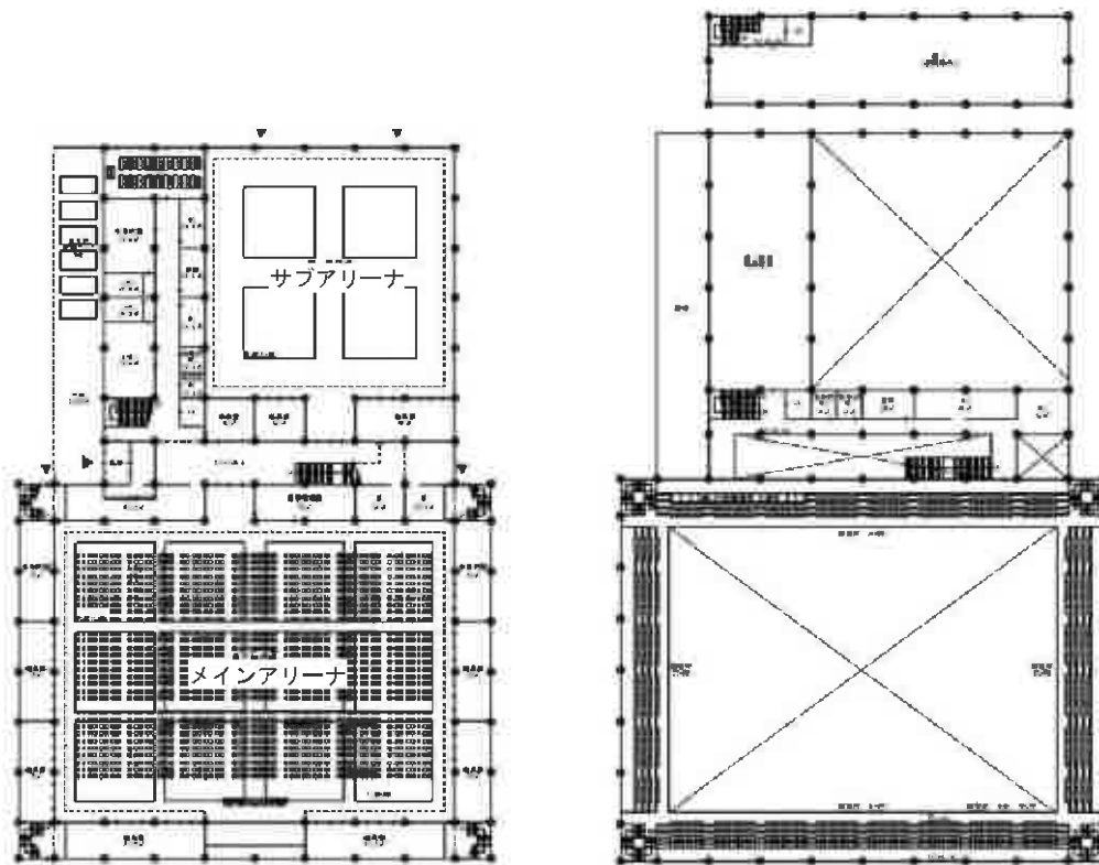
〔1F 平面図〕
