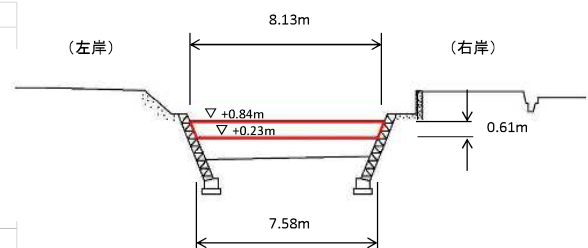
新津橋下流横断面図
