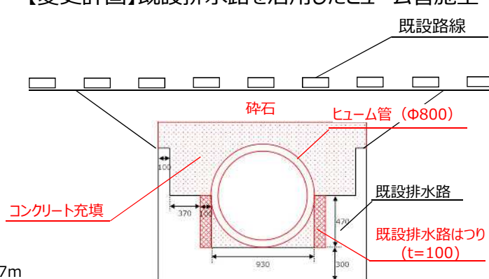
【変更計画】既設排水路を活用したヒューム管施工
