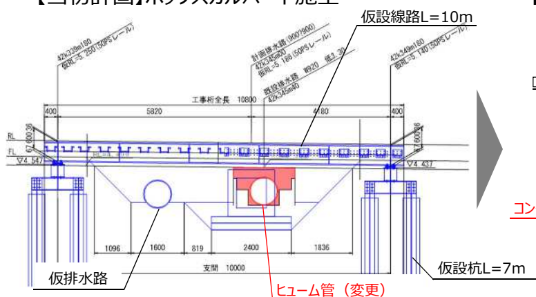
【当初計画】ボックスカルバート施工
