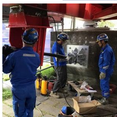
水管橋の耐震化工事（2022年度） 〔常光浄水場〕
