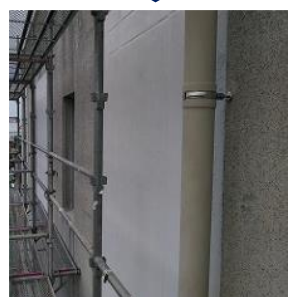
開口部閉塞によるポンプ場の耐震化 (2020 年度) [中田島団地雨水ポンプ場]
