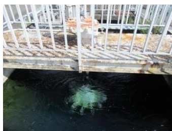
省エネルギー設備へ 更新予定の急速攪拌機 〔常光浄水場〕
