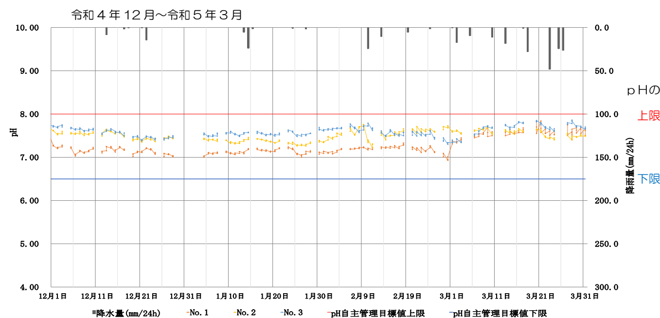
[水質調査結果（水素イオン濃度(pH)）_令和4年4月～令和5年3月]
