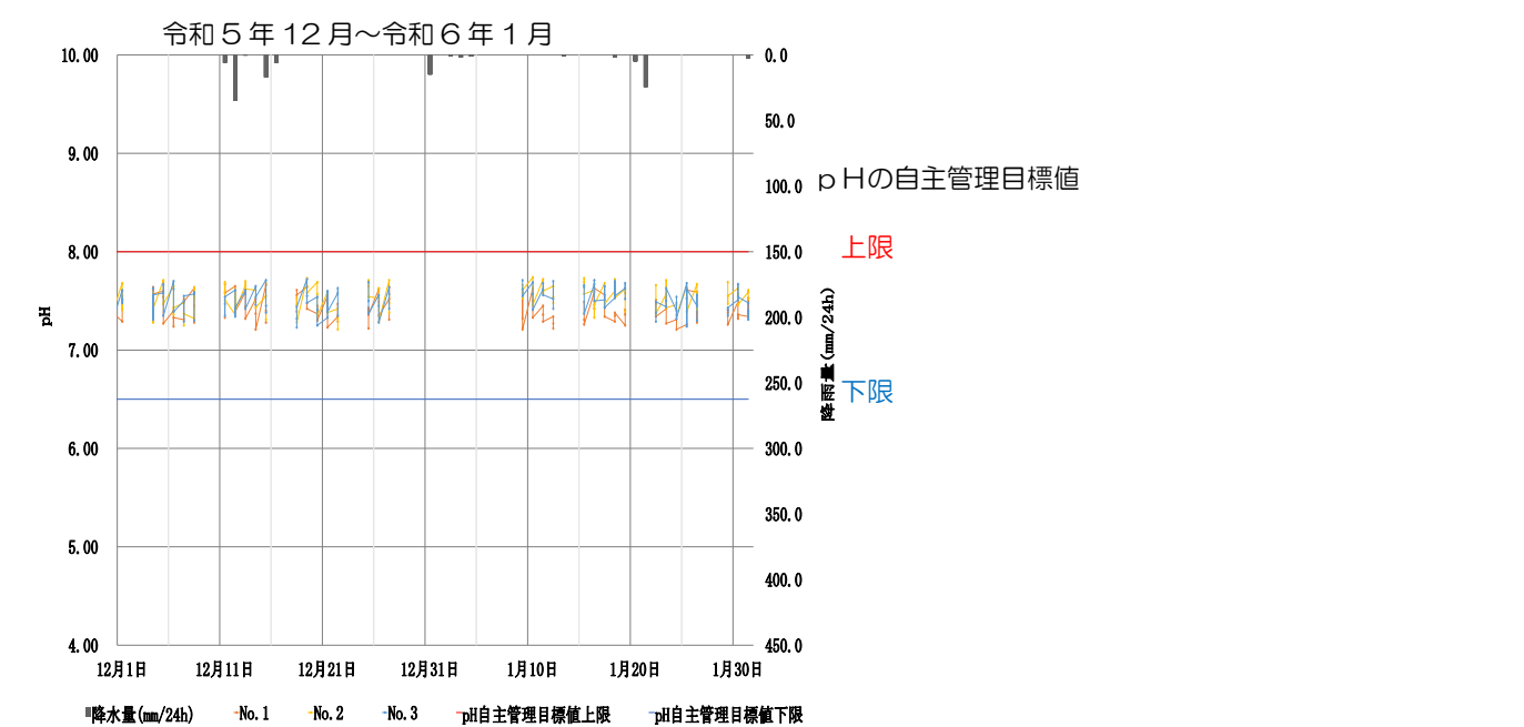
[水質調査結果（水素イオン濃度(pH)）_令和5年4月～令和6年1月]
