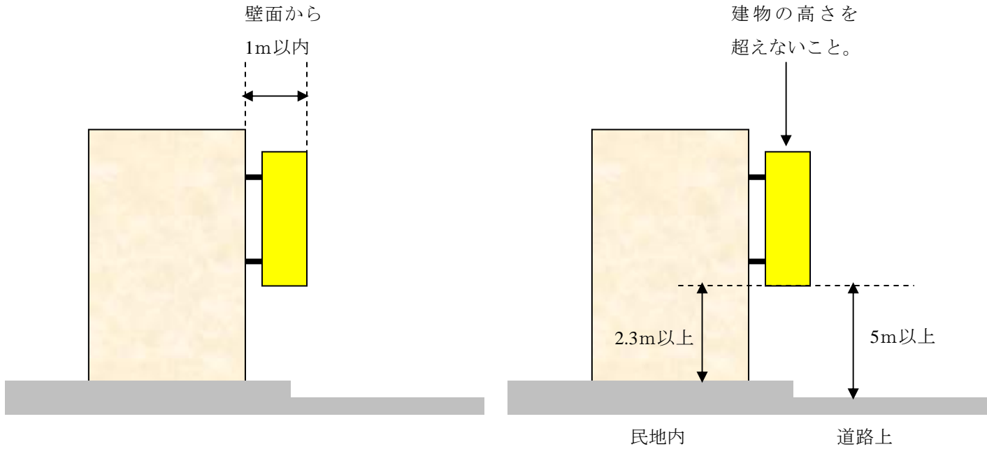
突き出し幅
