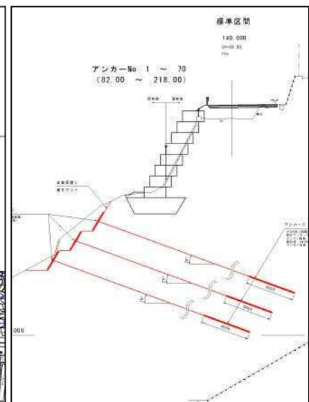
(標準横断面図)
