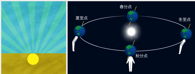
図1：日の出入りの瞬間の位置(太陽の上辺が地平線に接したとき)
