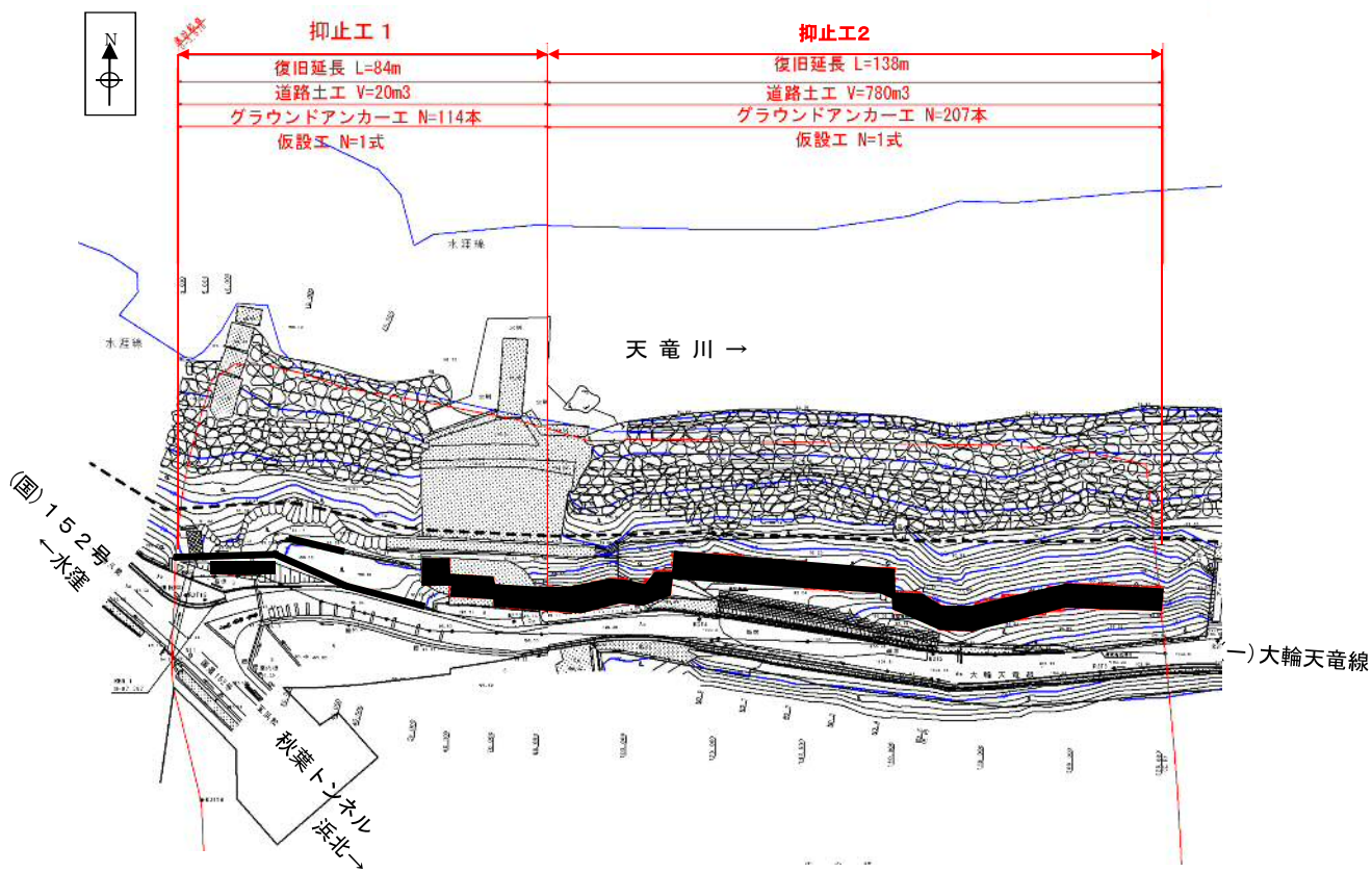
(計画平面図)
