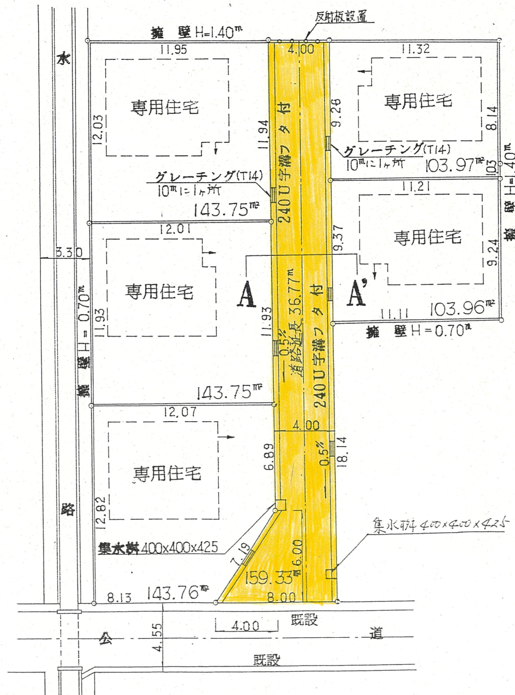
実測図 1:250
