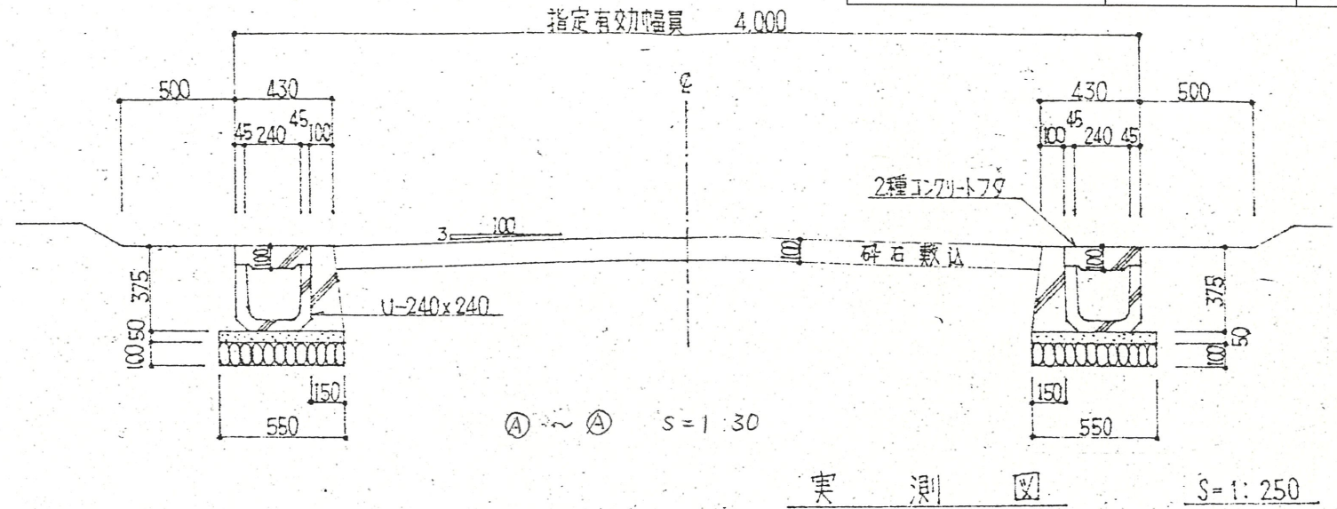
2 断面図
