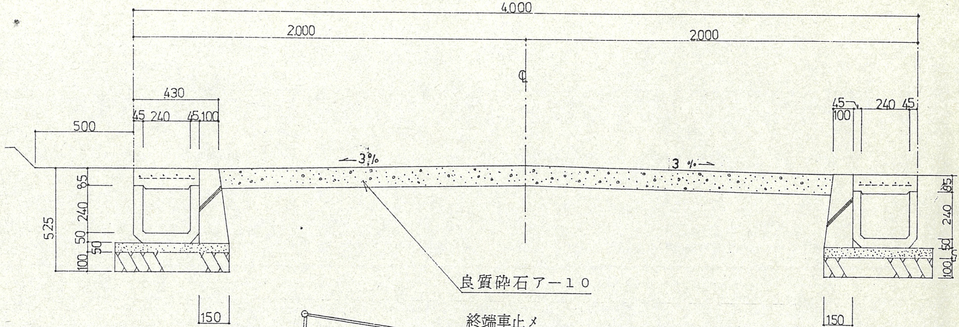
2 断面図 S=1/20
