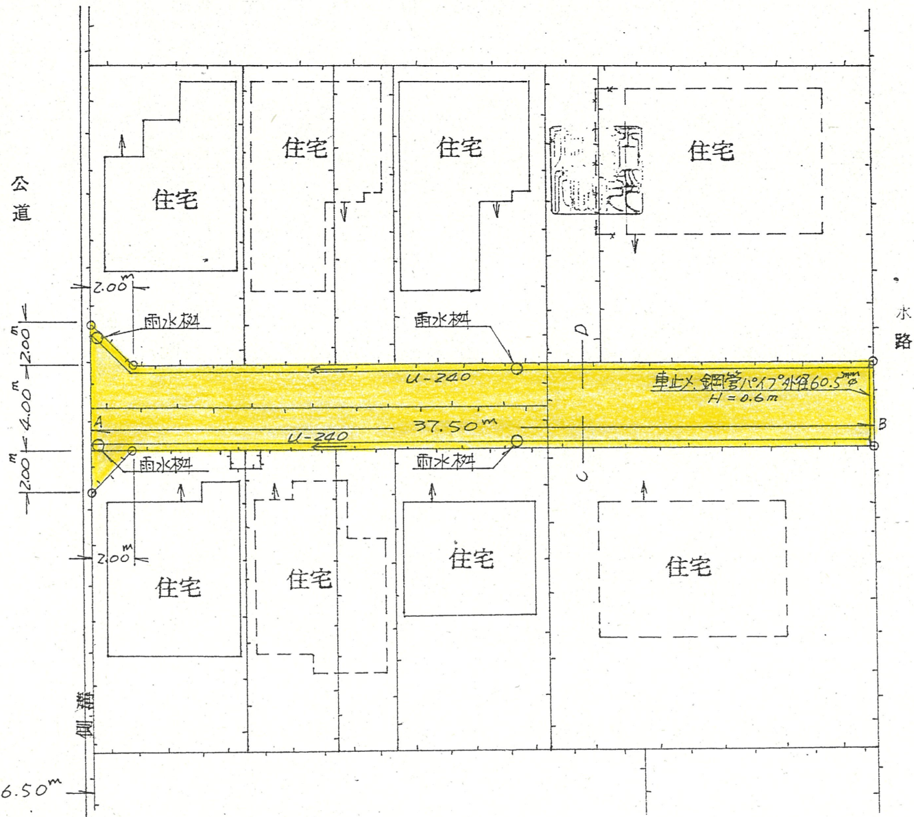
実測図 1/250
