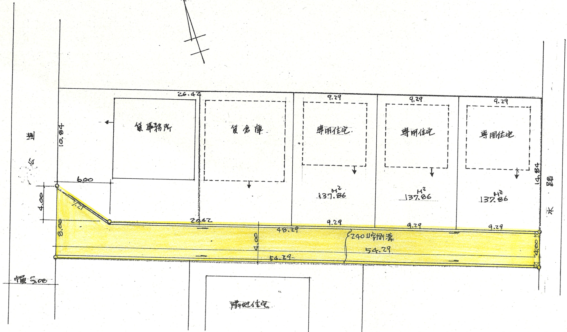
実測図 1/250
