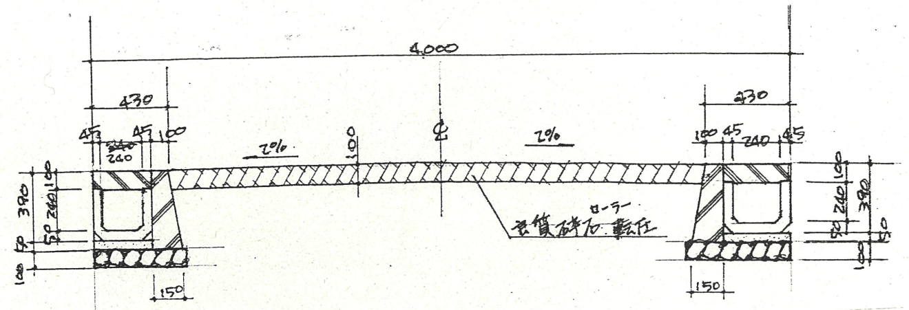
実測図 1/250
