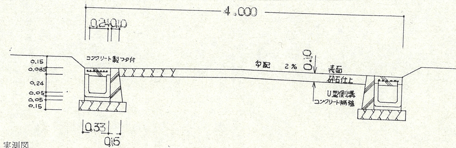
AA 断面図 1/30
