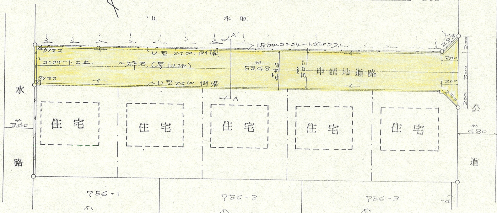
実測図 \frac{1}{300}
