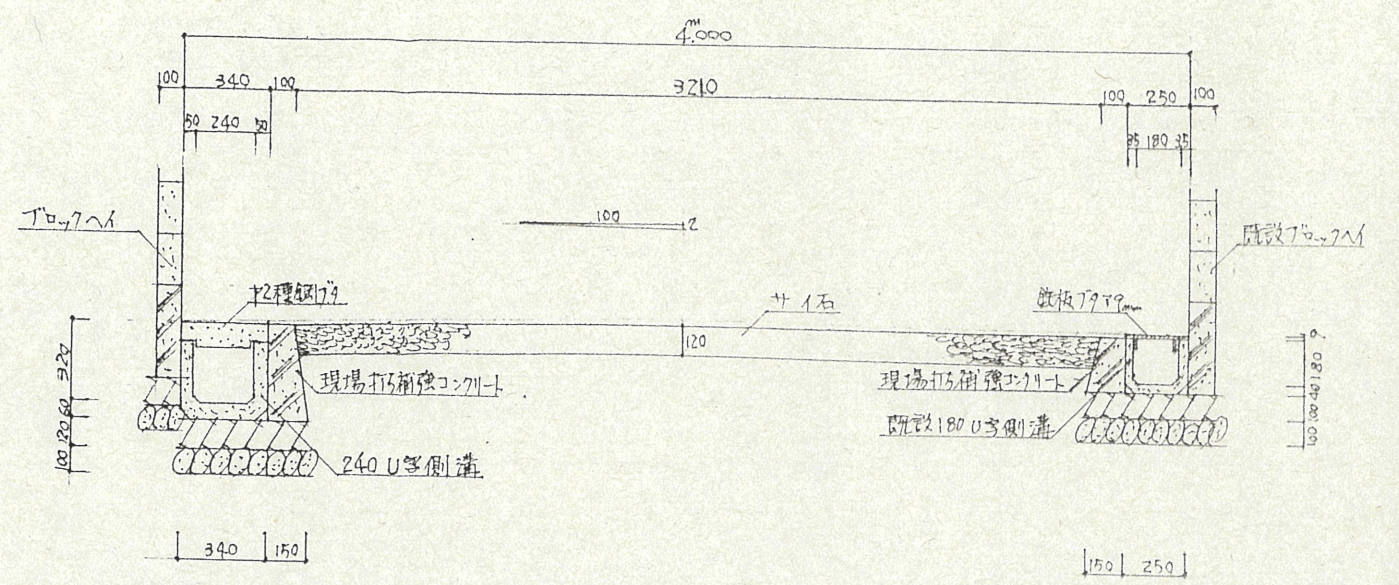
S-S' 断面図
