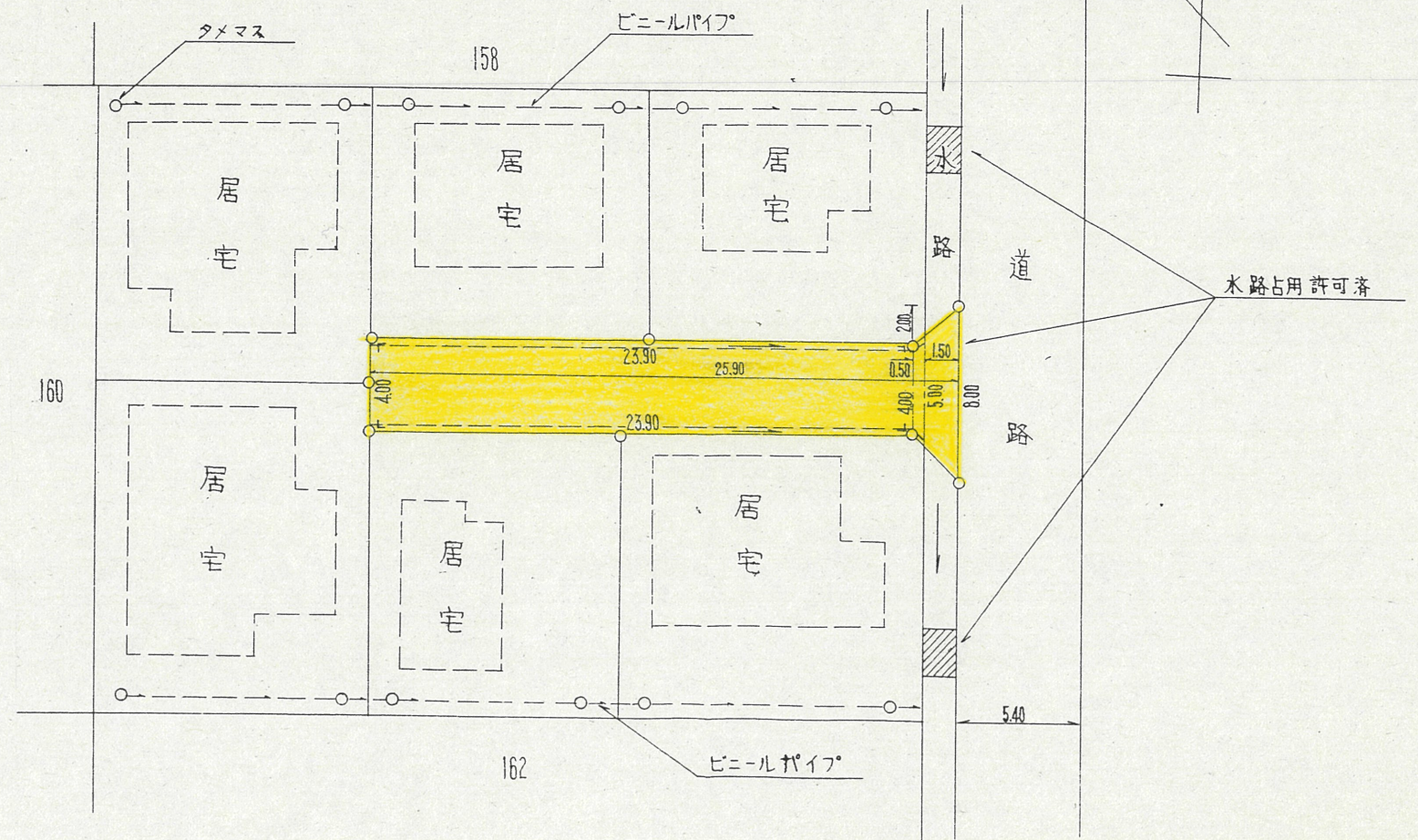
実測図 1/300
