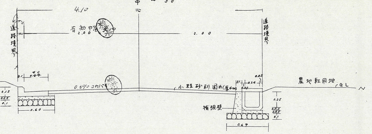
A.A 断面図 S 1/30
