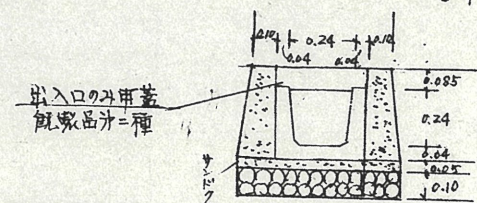
出入口断面図 S=1:30
