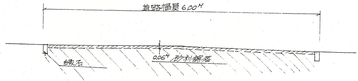
実測図 S 1/300
