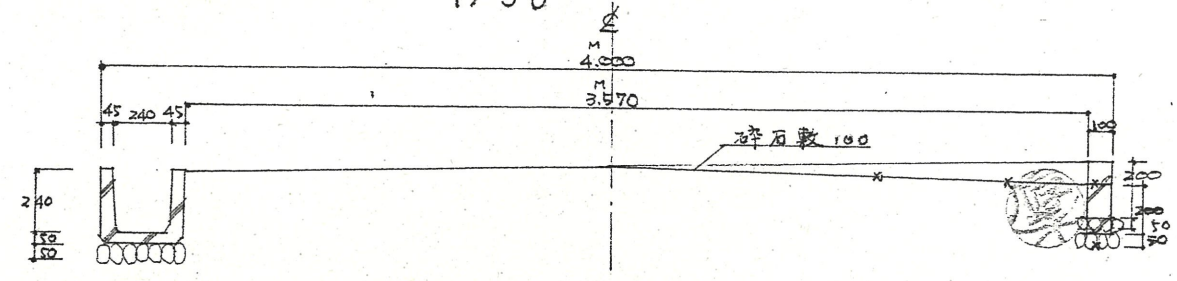
断面図 1/30
