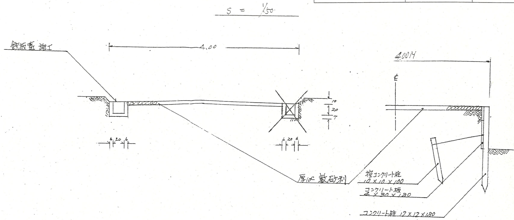
断面図
