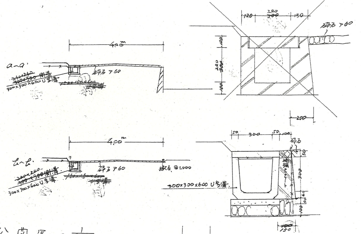
断面図 S 1/100
