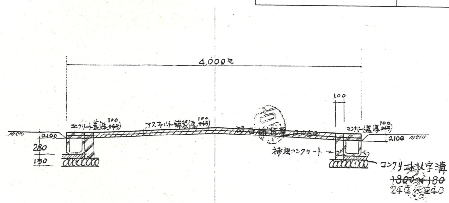
断面図 1/50
