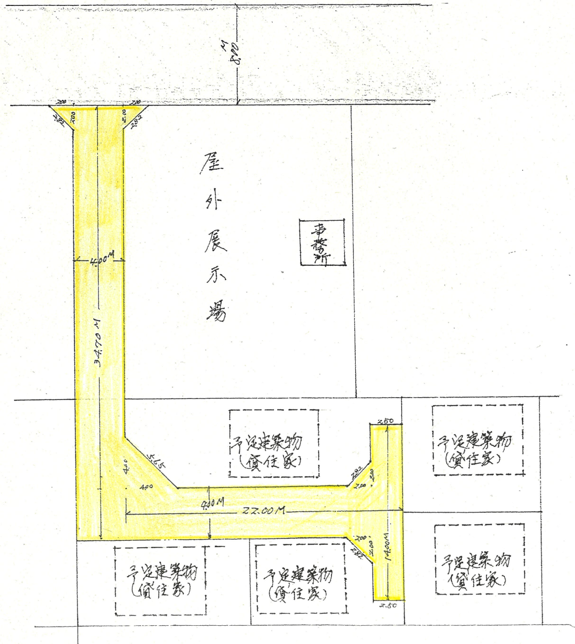
尺測図 S = 1/300
