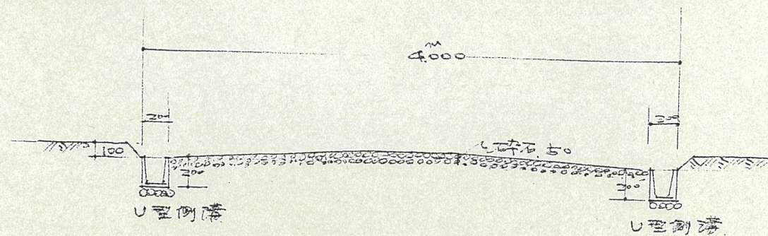
断面図 1/40
