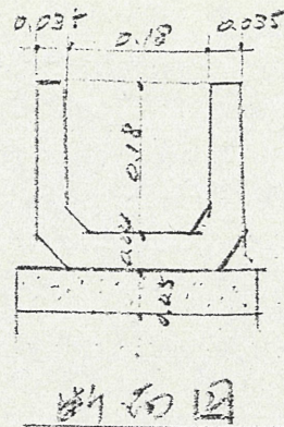
断面図 S=1/50
