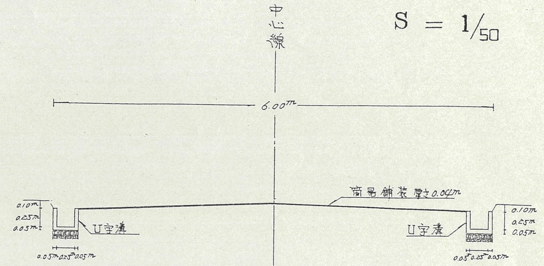
① 断面図
