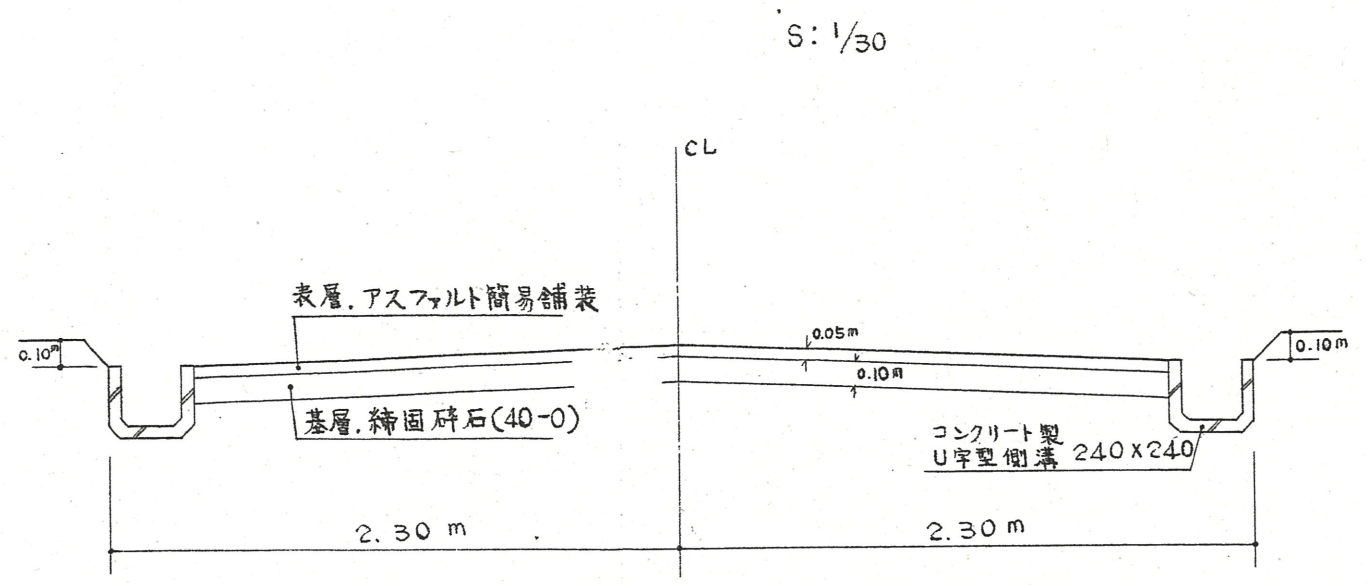
実測図
