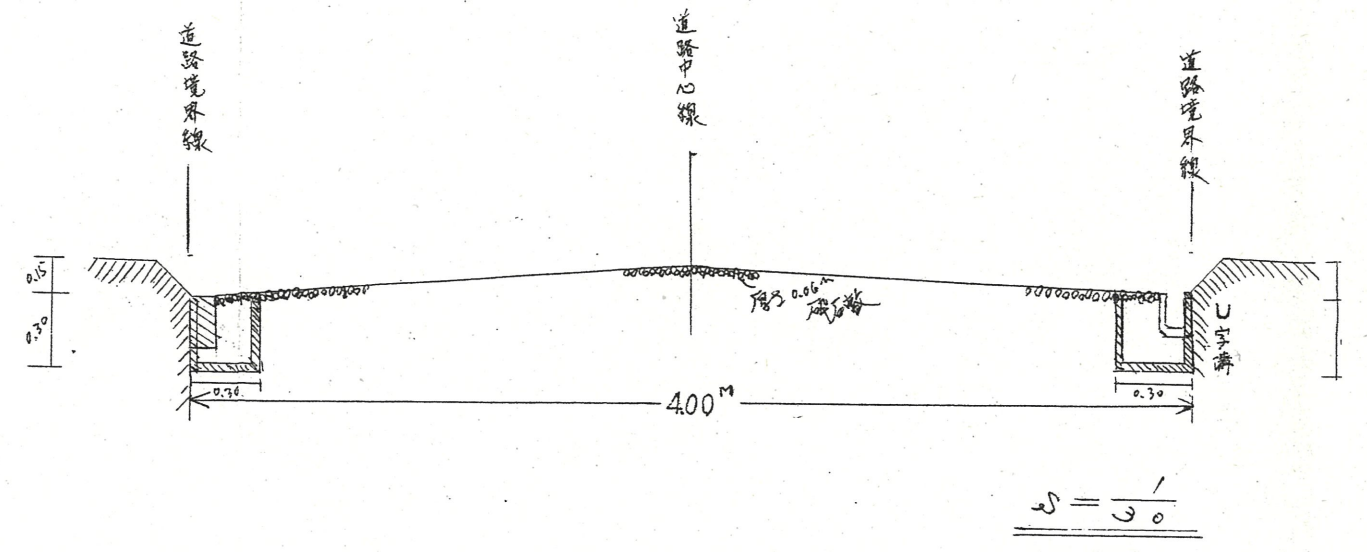
断面図
