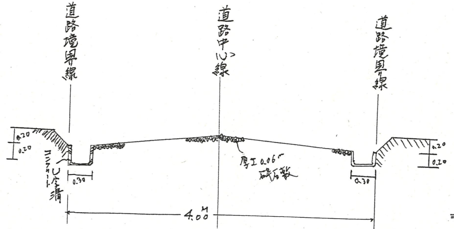
断面図 S = \frac{1}{50}
