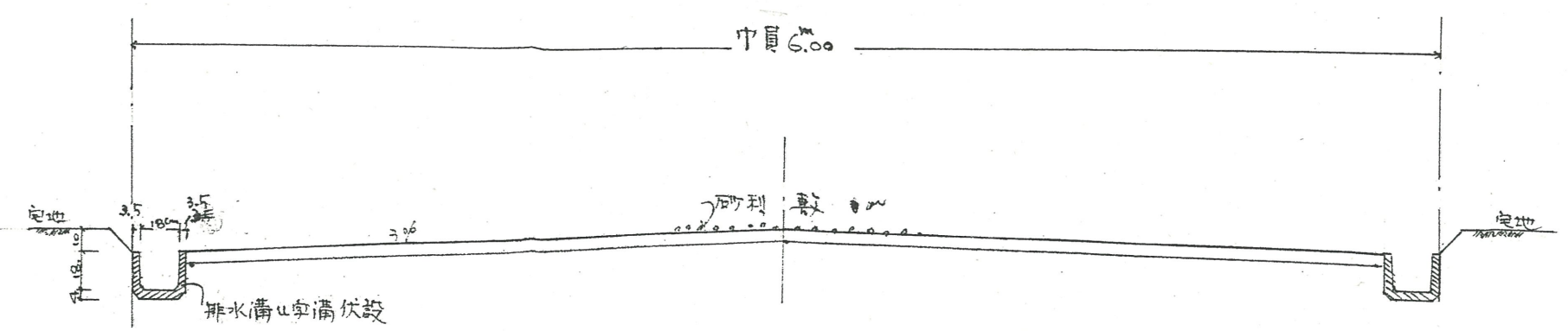
断面図 \frac{1}{30}
