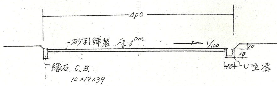
断面図 S:1:50
