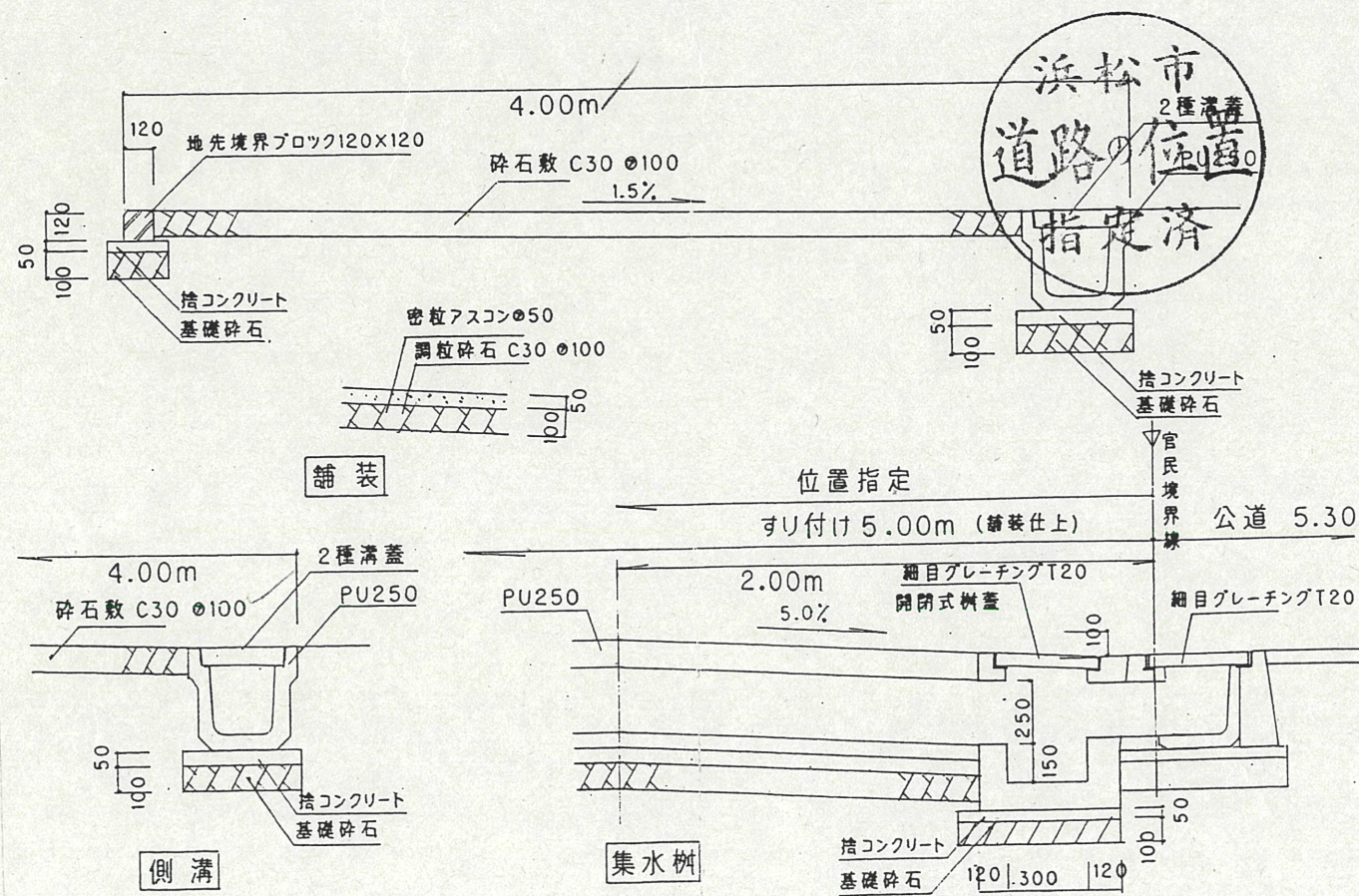
道路断面図 S=1/30
