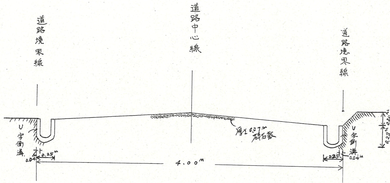
断面図
