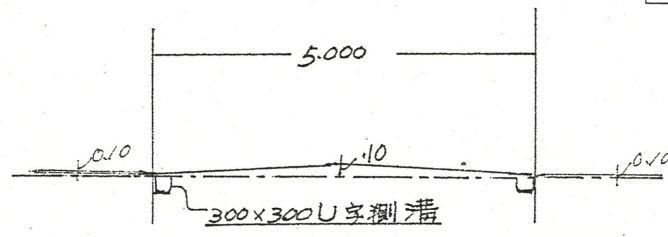
横断面図 1/60
