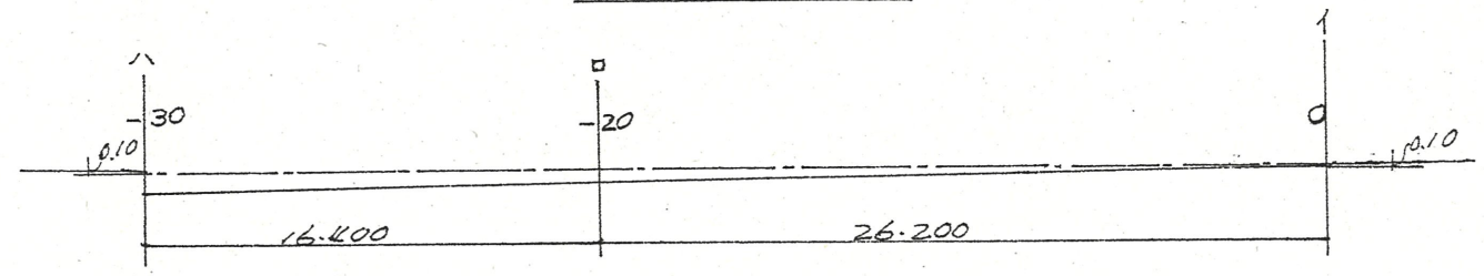
縦断面図 1/300
