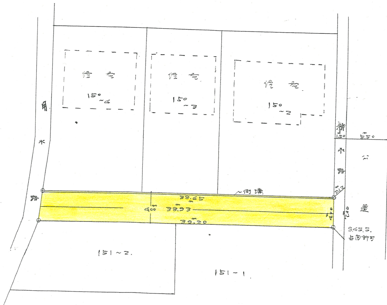
実測図 1/300
