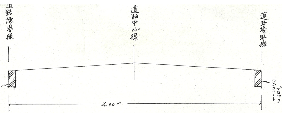
断面図 S = \frac{1}{30}
