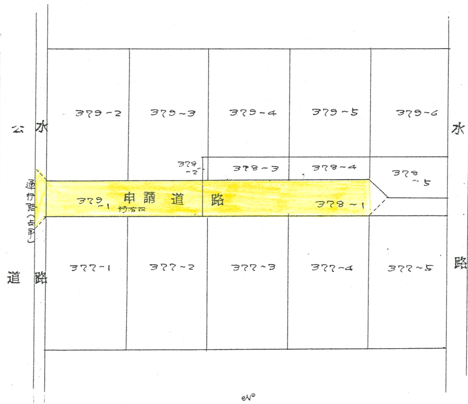
公図写 1/500
