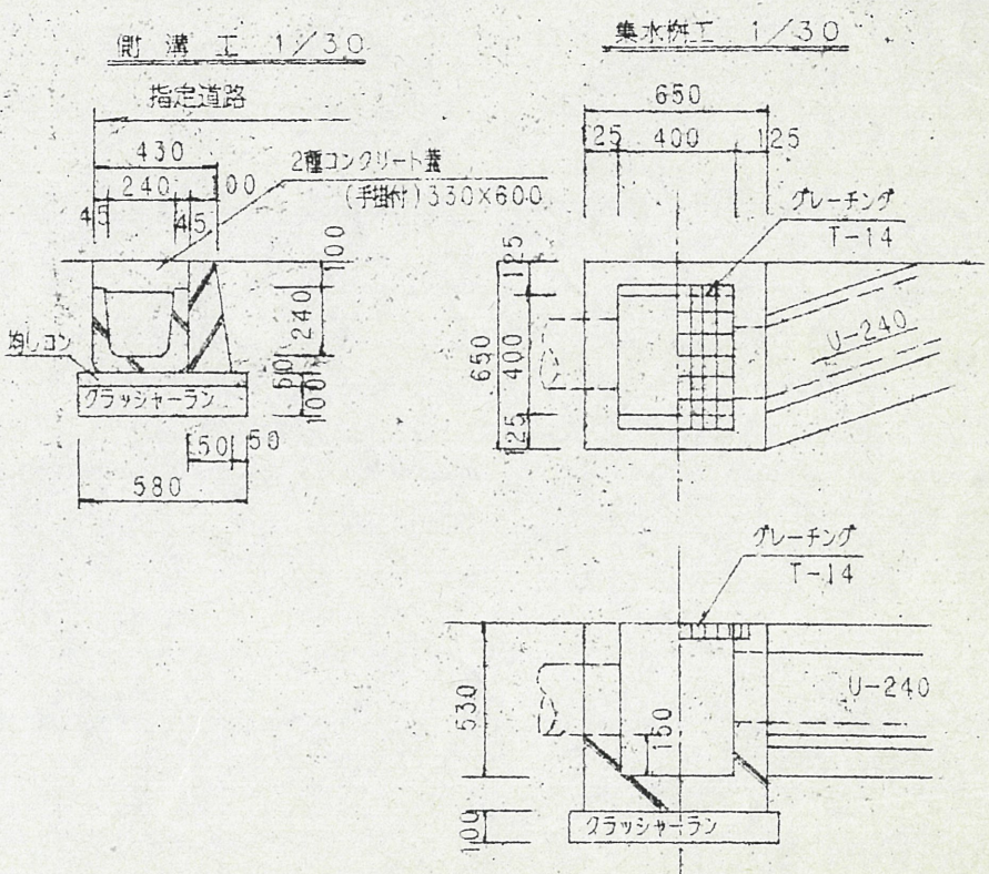
2 断面図
