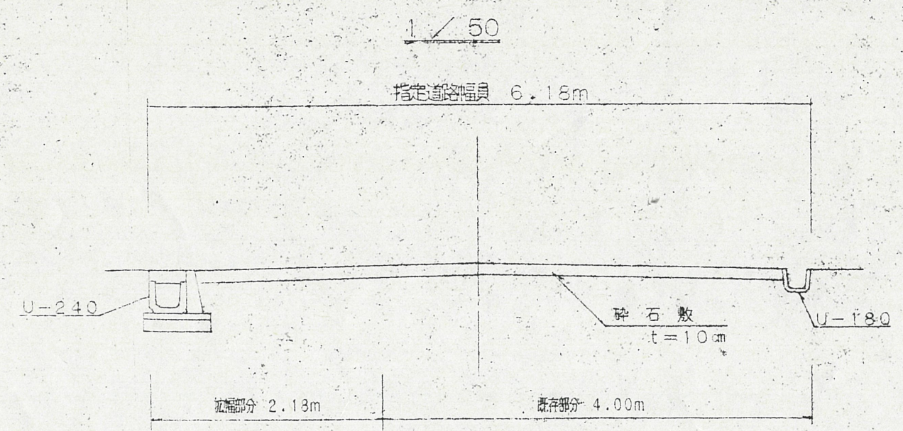
2 断面図
