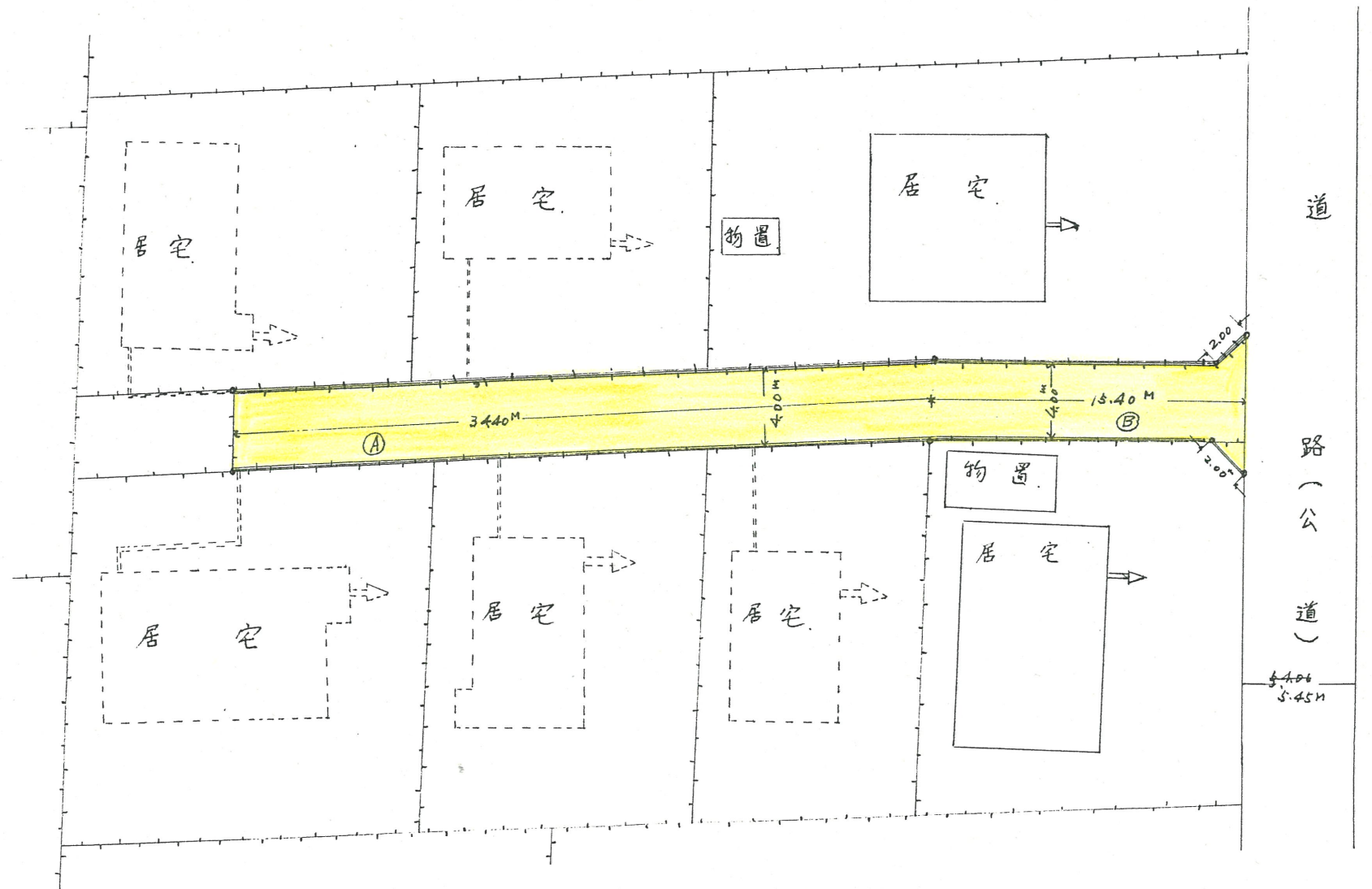
実測図
