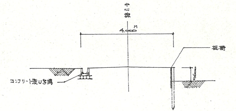
断面図 1:100
