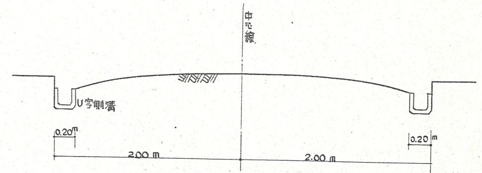
実 測 図 1/300
